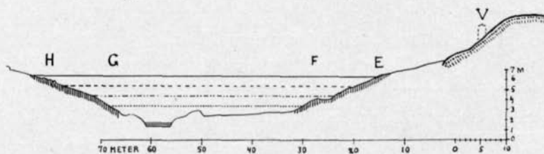
Fig. 4. Profil tvärs över Ramsundet och längs brofästena.
